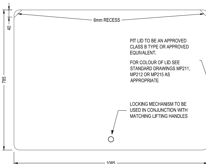
LID SCALE 1:10
